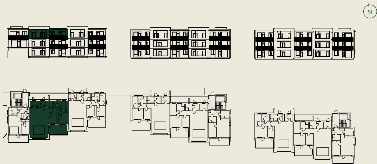
Etasjeplan og fasade sett fra sør
